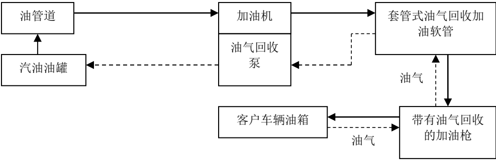
图 2-2 汽油加油及加油油气回收工艺流程示意图
