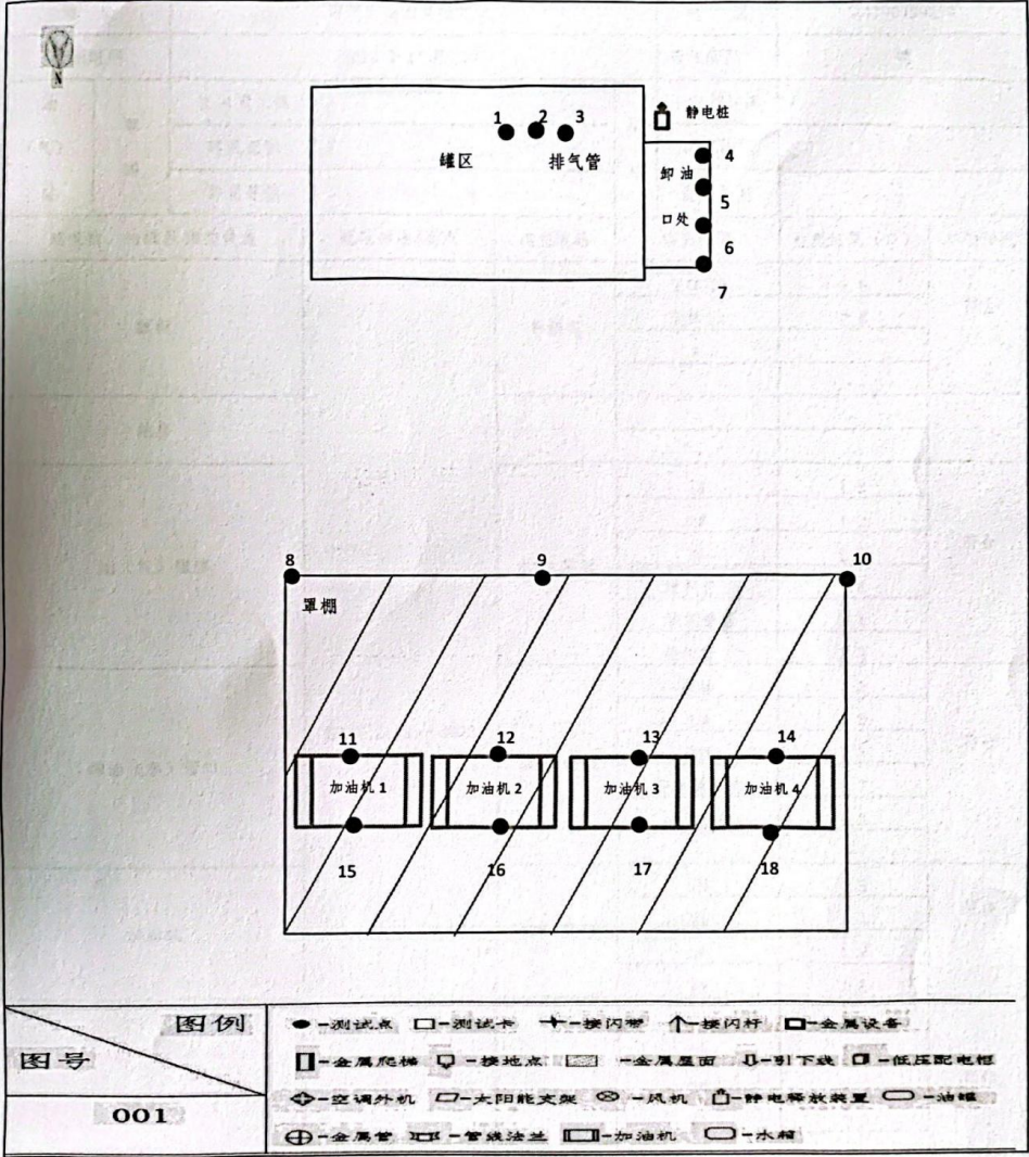
定期检测项目平面布置图
