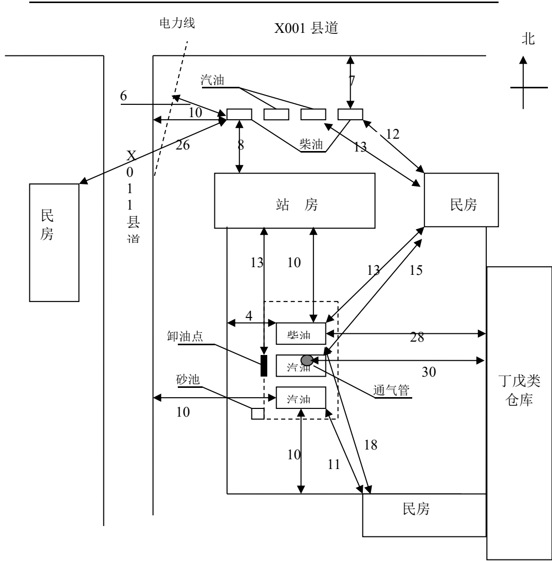
砀山县园艺场宾友加油站平面布置示意图
