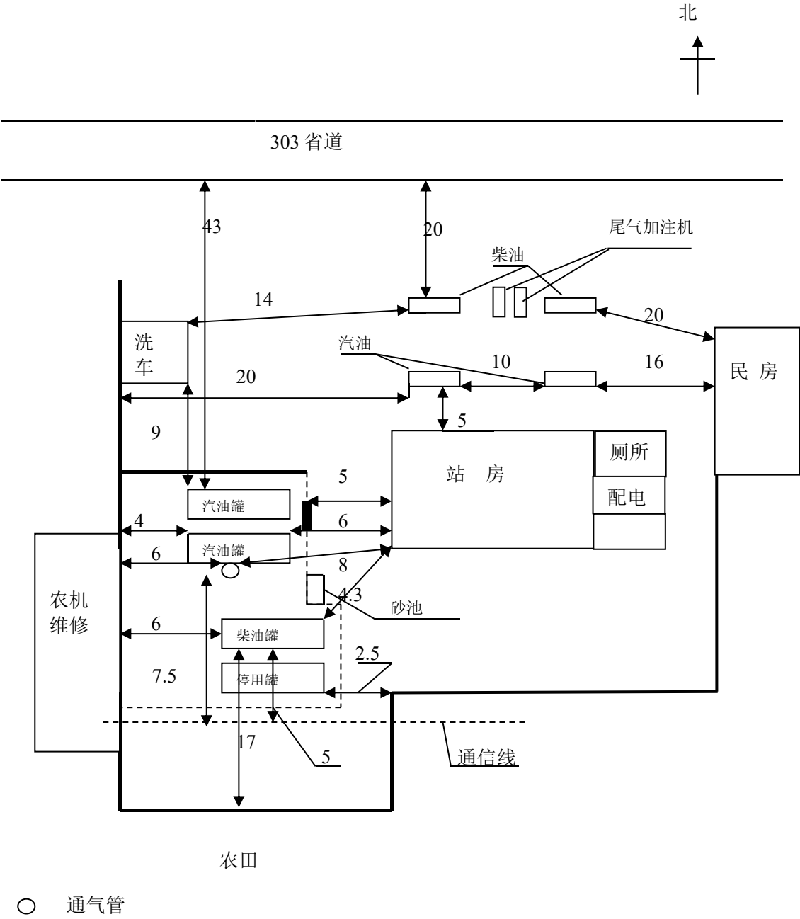
灵璧县娄庄镇东加油站平面布置图
