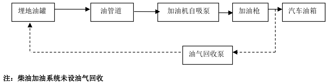
图 2-3 加油工艺流程示意图
