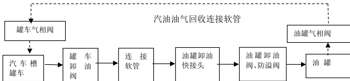
图 2-2 汽油卸油工艺流程示意图
