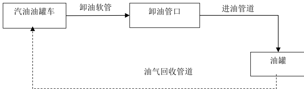
图 2-1 汽油卸油工艺框图
