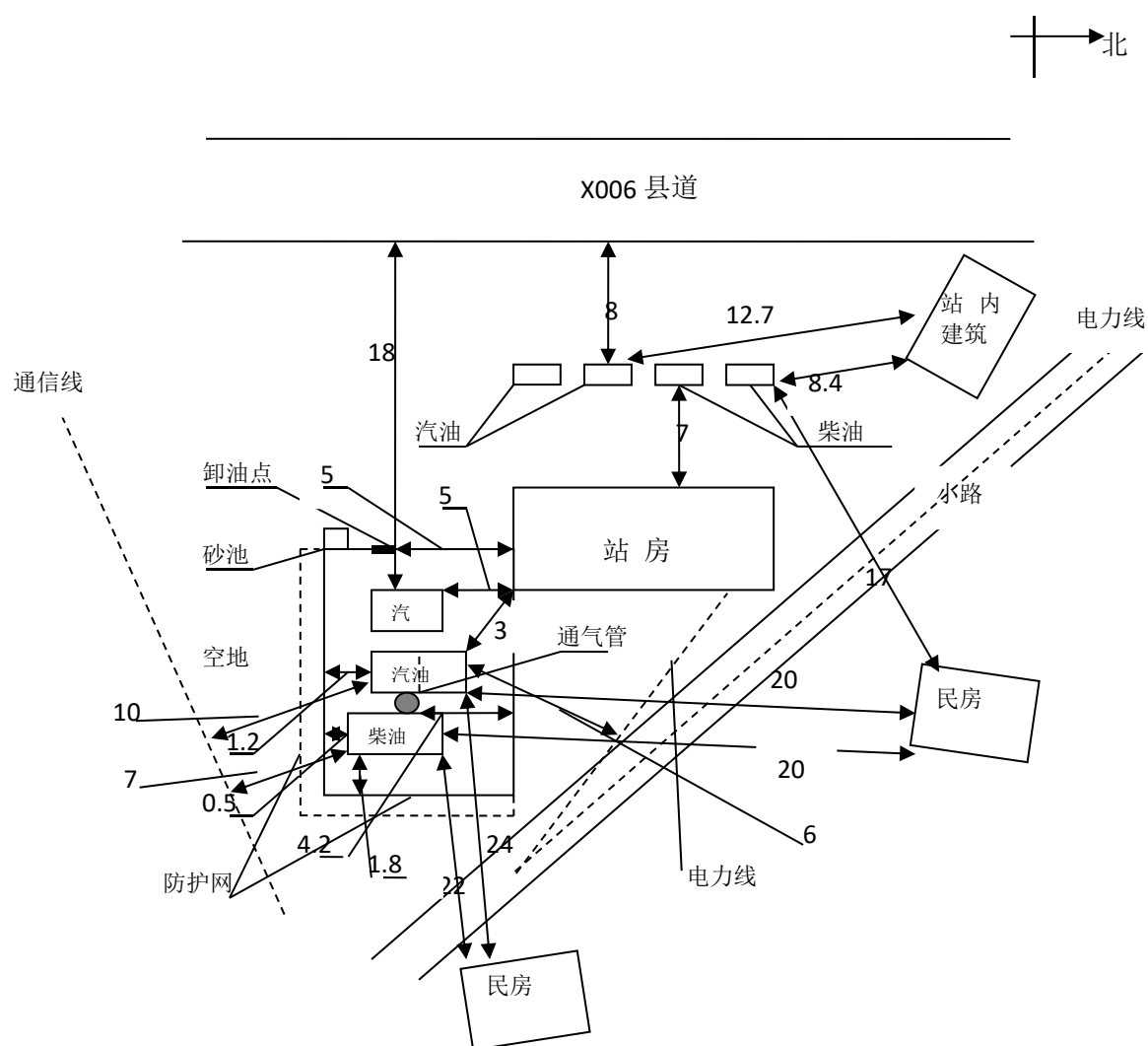
附件 10 加油站周边环境及平面布置图
