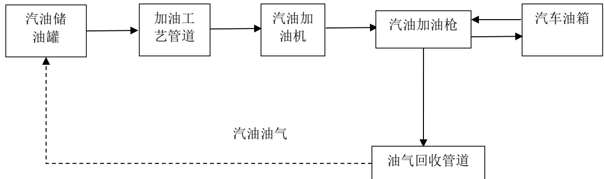
图 2-4 汽油加油工艺框图
